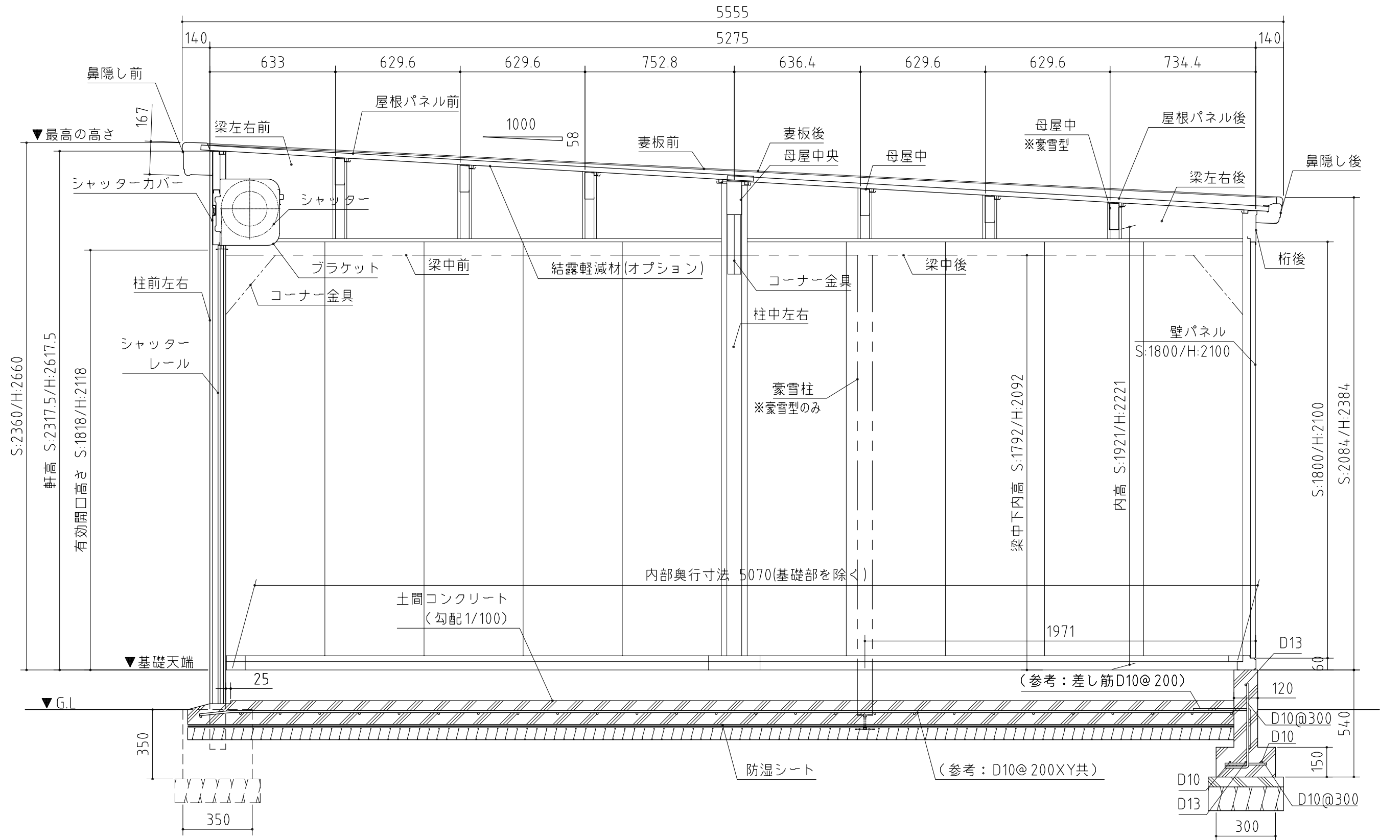
断面図(側面) <縮尺> S=1/20 ~一般型・豪雪型~ 機種名 GRN- 2652S・SL・H・HL, 3152S・SL・H・HL 3652S・SL・H・HL
